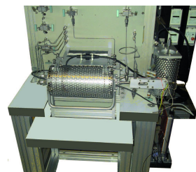
高温相对渗透率系统 RPS-HT
