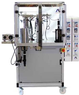
气体加载系统 GLS1500
